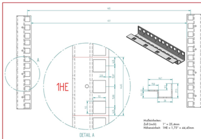
■ SCHNITTANSICHT DER VERTIKALEN 19"-PROFILSCHIENEN
