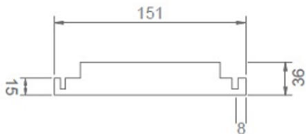
widok z boku / side view
