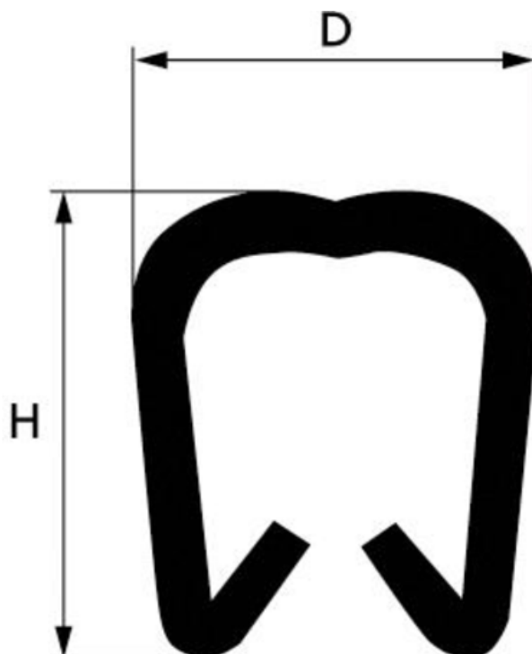
LAPP INEL DE MARCARE PC 20/7
