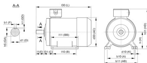
Рисунок 1. Размеры двигателей монтажного исполнения IM 1081.
