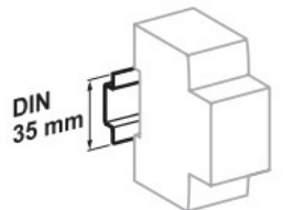
Fixare pe șină DIN de 35 mm.
